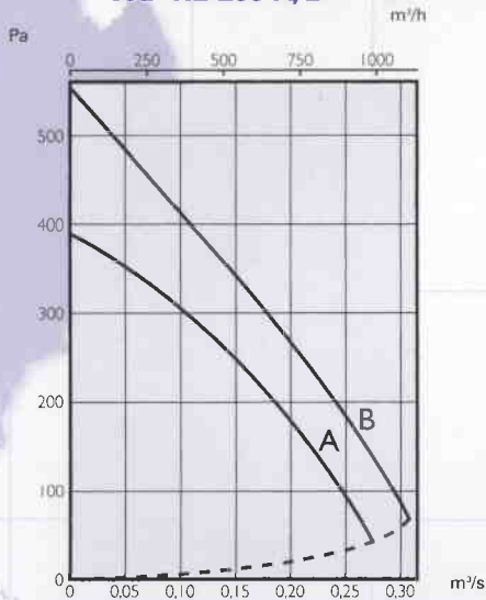
WD-KE 200 A/B
