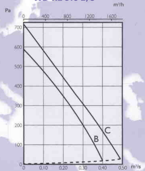
WD-KE 315 B/C
